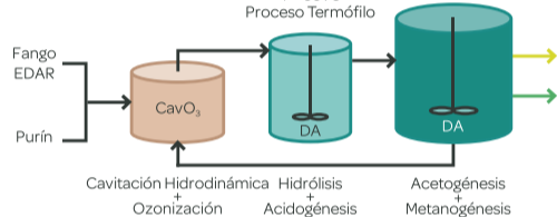
Fig.2 - Proceso de Digestión Anaerobia STO3RE
