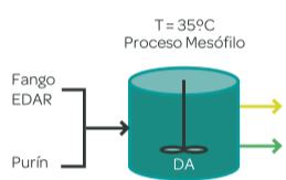
Fig.1 - Proceso de Digestión Anaerobia CONVENCIONAL
